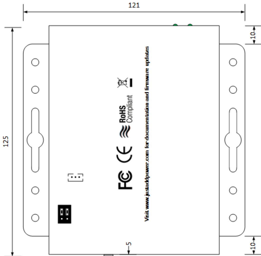
505PoE Bottom
